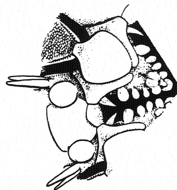
Figure 18. Ophioneis surbrachyplax .
