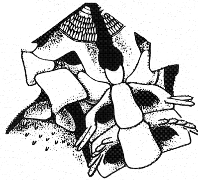
Figure 27. Ophiothrix rudis .
