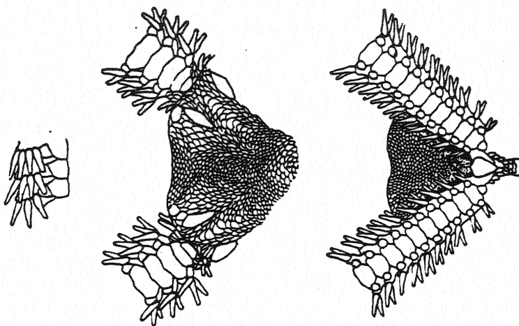
Figure 18. Ophioneis surbrachyplax .
