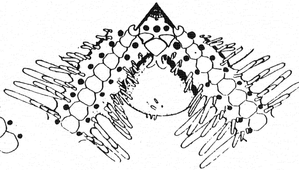
Figure 27. Ophiothrix rudis .
