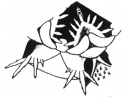
Figure 32. Ophiacantha rhachophora .
