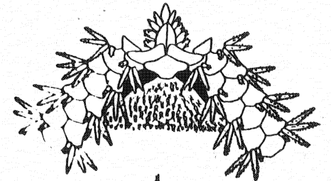
Figure 32. Ophiacantha rhachophora .
