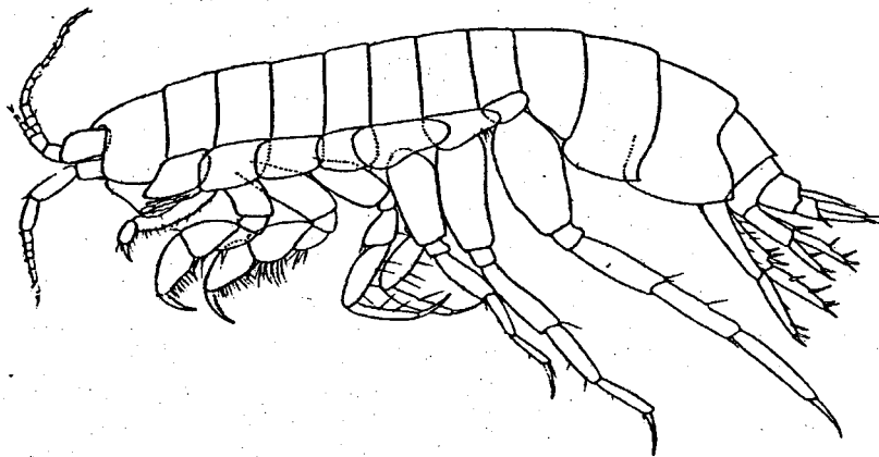
Fig. 3. Pardaliscella symmetrica n. sp. Male, 3mm, station 4951.
